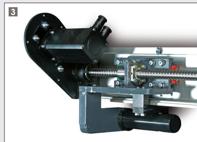
Nauwkeurige sturing van de parallelaanslag met een kogelomloopspindel en lineaire geleidingen
